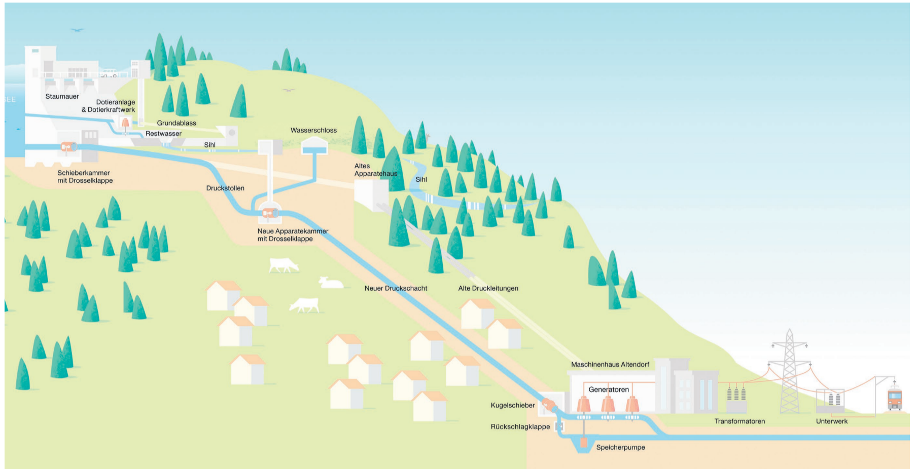
In den Schlägen in Egg bei der Staumauer des Sihlsees wird ein neues Dotierwerk gebaut, welches kühles Tiefenwasser aus dem See in die Sihl abgibt.
